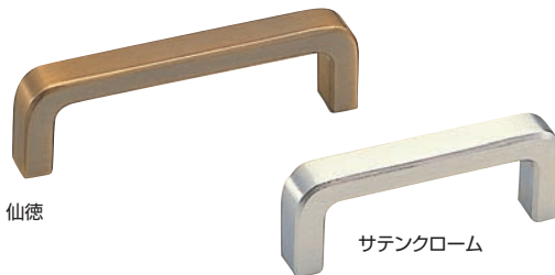
HB-50 真チユウ公団型角形一文字取手 (真チユウ/ISO4×28)
