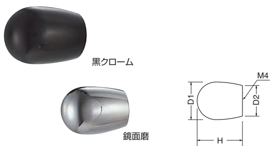
ST-68 ステン風船ツマミ (ステンレス/4×28)
