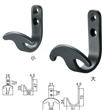
CF-12 イカリフック (鉄)
