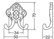
CB-22 ツインフック (真チュウ/3.1×22)
