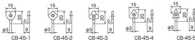
CB-45 ラッキーフック (真チュウ/皿φ2.4×13)
