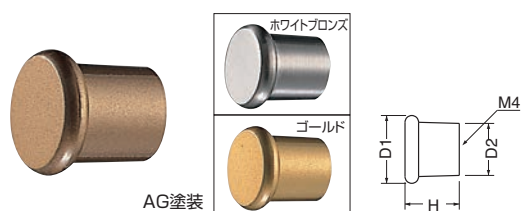
KZ-10 オレゴンツマミ (亜鉛合金/ISO4×28)
