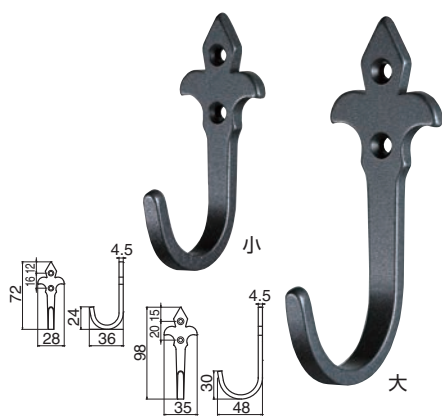
CF-17 アンティークフックアイリス (鉄/3.1×16)
