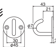
ST-267 ステン丸座フックU形 (ステンレス/A4×25)
