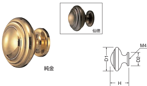
KB-15 ナタリーツマミ (真チュウ/ISO4×28)
