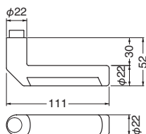
SL-324 - R - GF - クローム R座空錠付セット価格 13,950
