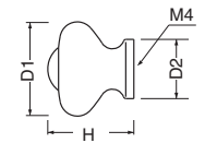
KC-7 ボヘミアツマミ (自然木+真チュウ/ISO4×28)
