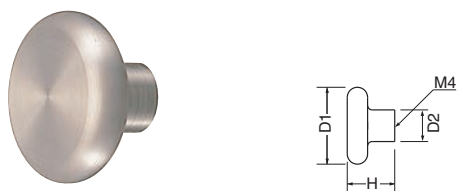
A-44 マッシュルームツマミ (アルミ/ISO4×28)
