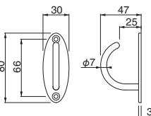
ST-264 ステンダエンフックR形 (ステンレス/A4×25)
