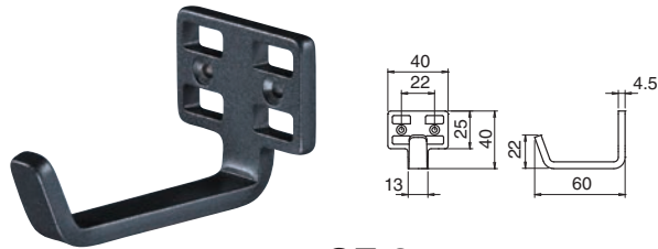
CF-24 四角フック (鉄/3.1×22)
