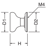
KB-20 エポックツマミ (真チュウ+エポキシ/ISO4×28)
