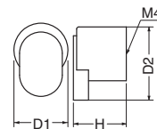
KB-54 ジュネーブツマミ (真チュウ/NL4×28)
