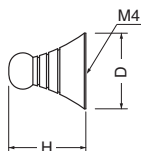
KB-62 ネオンツマミ (真チュウ/ISO4×28)
