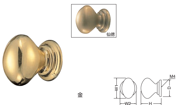
KB-49 ブルボンツマミ (真チュウ/ISO4×28)
