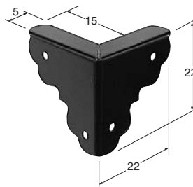
LA-10 飾り三ツ折 黒 135 22×22×22 400個入
