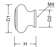
KW-19 エジンバラツマミ (自然木/ISO4×28)
