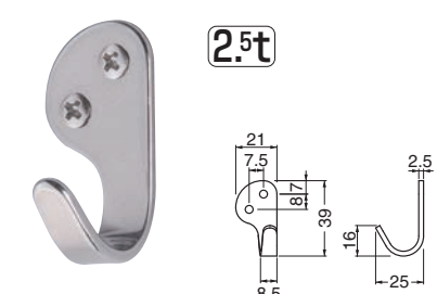
ST-255 ステンQ形フック (ステンレス/低頭A3×16)
