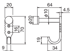
CF-28 ブルゴス帽子掛 (鉄/3.1×22)
