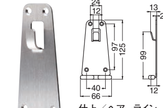
FEX-4 ステン消火器フック台形 (ステンレス+エラストマー/A4×25)
