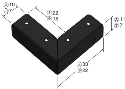
LA-8 角金具 黒 ③33×33 135 ④22×22 135 600個入
