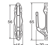
CZ-7 マーチン房掛 (亜鉛合金/3.1×16)
