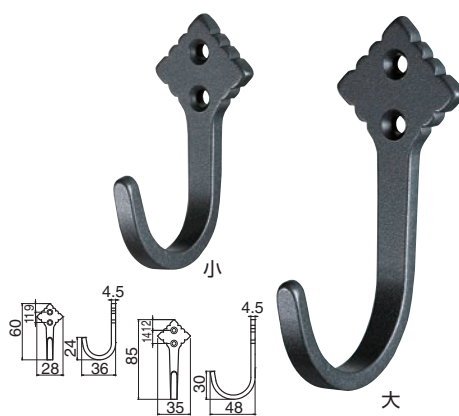
CF-18 アンティークフックダイヤ (鉄/3.1×16)
