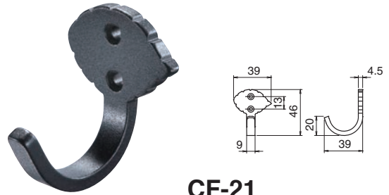
CF-21 リーフフック (鉄/3.1×16)
