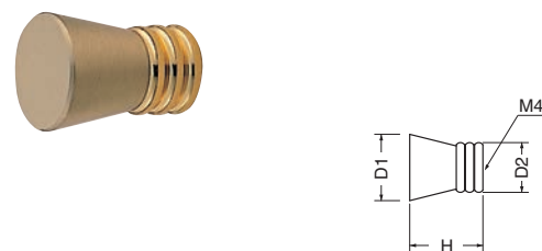
KB-75 シプレツマミ (真チュウ/ISO4×28)
