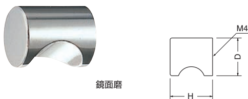
ST-11B ステンニューカットツマミ (ステンレス/NL4×28)
