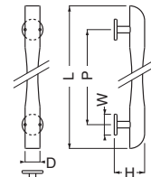
No.22 ウッド平丸取手 木ネジ止め (横溝+真チュウ/3.1×22)
