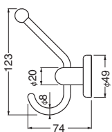
CB-39 プラネット帽子掛 (真チュウ/A4×30)
