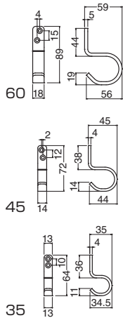
ST-210 ステンビームフック (ステンレス/A4×25)
