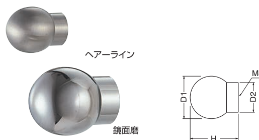
ST-73 ステンモナリザツマミ (ステンレス/4×28)
