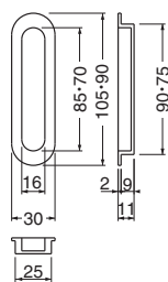
MW-17 ウッド小判戸引手 (積層)
