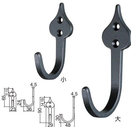
CF-15 アンティークフックスペード (鉄/3.1×16)
