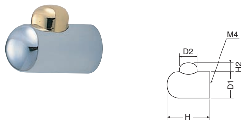
KB-82 デュオツマミ (真チュウ/ISO4×28)
