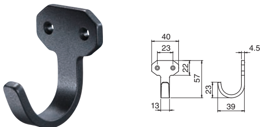
CF-26 八角フック (鉄/3.1×16)
