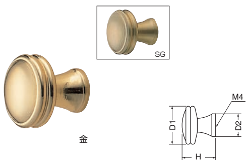
KB-77 レイナツマミ (真チュウ/ISO4×28)
