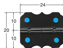
LA-67 飾り立丁番90度 黒 180 24×(10+10) 600個入
