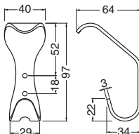
ST-281 ステンダ・ヴィンチ帽子掛W形 (ステンレス/低頭A4×25)
