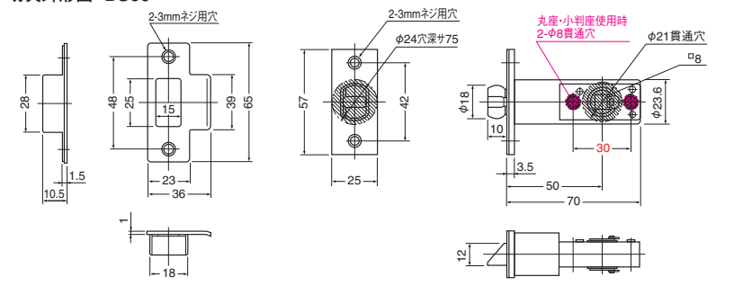
切欠外形図 BS50
