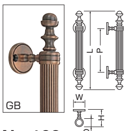
No.102 モーゼル取手 木ネジ止め (真チュウ/3.1×22)
