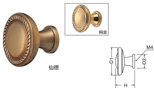
KB-14 ルーキーツマミ (真チュウ/ISO4×28)
