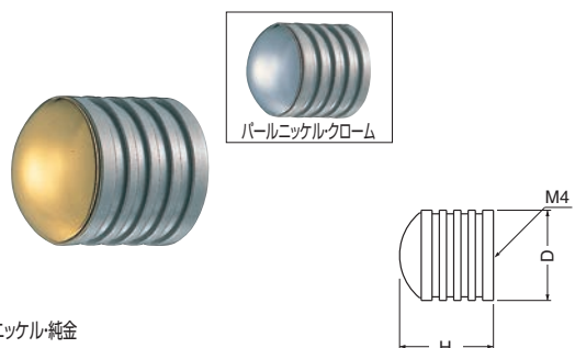
KB-101 パイロットツマミ (真チュウ/ISO4×28)
