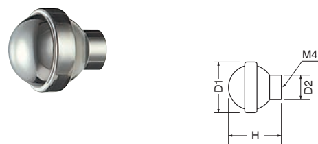
ST-74 ステンワールドツマミ (ステンレス/4×28)
