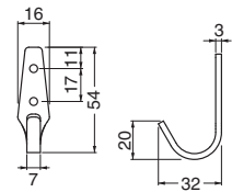
ST-261 ステンシルビアフック (ステンレス/低頭A3×16)
