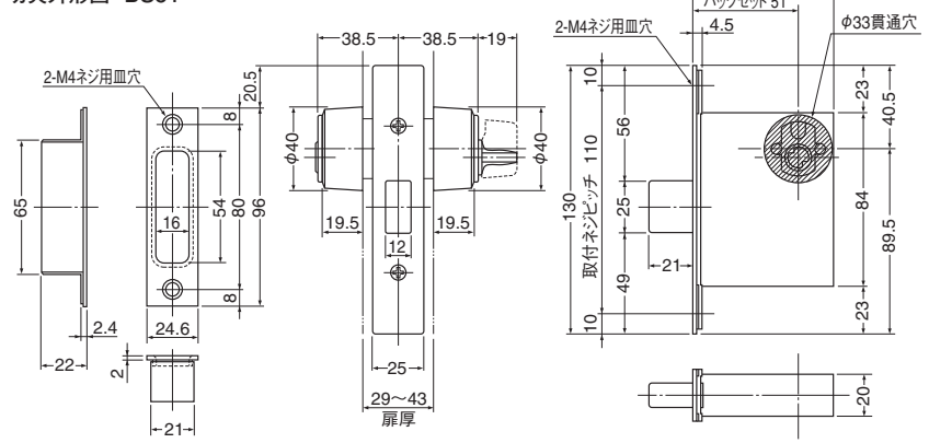
切欠外形図 BS51
