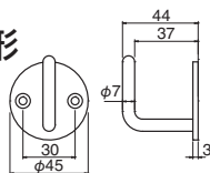
ST-267 ステン丸座フックU形 (ステンレス/A4×25)
