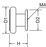
ST-60 ステンシスターツマミ (ステンレス/4×28)
