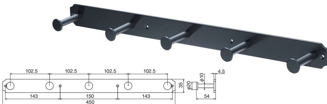
CF-36 ヨハネスフック五連 (鉄/3.1×22)
