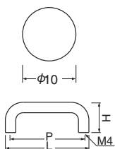
HB-59 真チユウ10φ丸棒ハンドル (真チユウ/ISO4×28)
