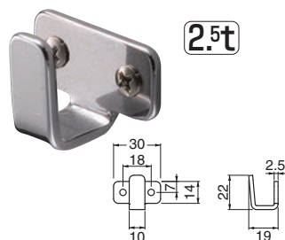
ST-253 ステンT形フック (ステンレス/低頭A3×16)
