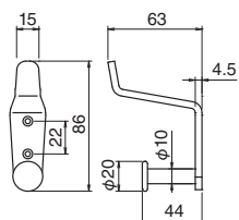
CF-31 ロベルト帽子掛 (鉄/3.1×22)
