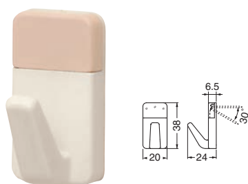
Iピンタイプ ※Iピンはペンチで簡単に抜けます。 C-181 アソートフック (ABS/ステンレス釘φ1.3×25)
