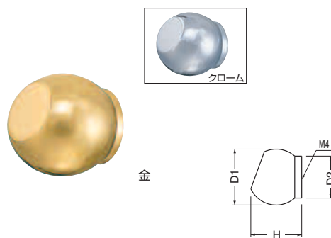
KB-103 レザンツマミ (真チュウ/ISO4×28)
