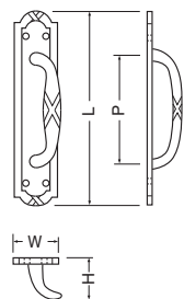
No.11 スパニッシュ座付取手 木ネジ止め (真チュウ/3.5×25)
