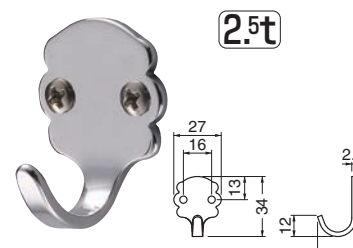
ST-257 ステンウェーブフック (ステンレス/低頭A3×16)
