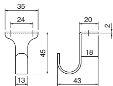
ST-91 トップフック (ステンレス/Ⅲ⊕3.5×25)
