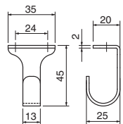
ST-91 トップフック (ステンレス/Ⅲ⊕3.5×25)
