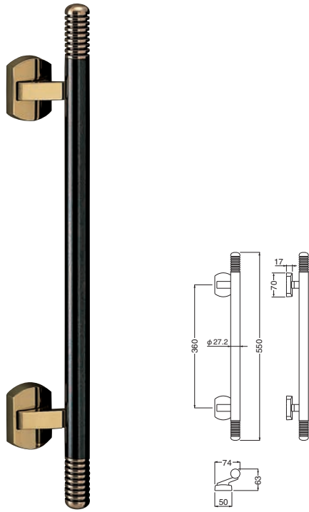
SPP-4 ベガ (真チュウ)
