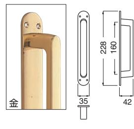
No.150 クラーク座付取手 木ネジ止め (真チュウ/3.5×25)
