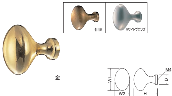
KB-34 フットボールツマミ (真チュウ/ISO4×28)
