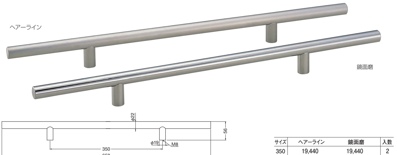
ST-38 ステン22φ丸棒ハンドル (ステンレス/8×30)
