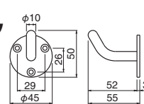
ST-56 ステン丸棒フック (ステンレス/A4×20)
