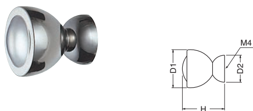
ST-71 ステンテ일러ーツマミ (ステンレス/4×28)
