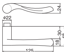
SL-17 - R - GF - シルバー R座空錠付セット価格 13,000
