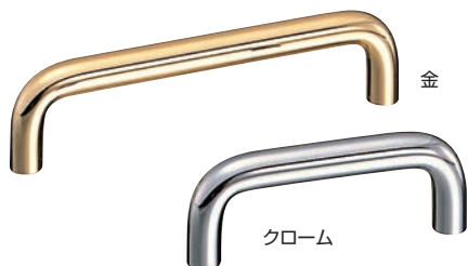
HB-59 真チユウ10φ丸棒ハンドル (真チユウ/ISO4×28)
