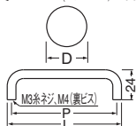
ST-100B ステン100番丸棒ハンドル裏ビス (ステンレス/ISO4×28)
