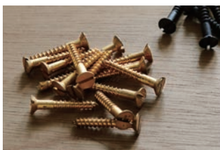
真鍮 皿木ねじ3.5×25(マイナスネジ)
