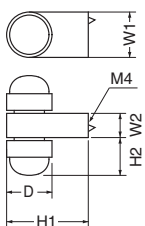
KB-71 パクスツマミ (真チュウ/ISO4×28)
