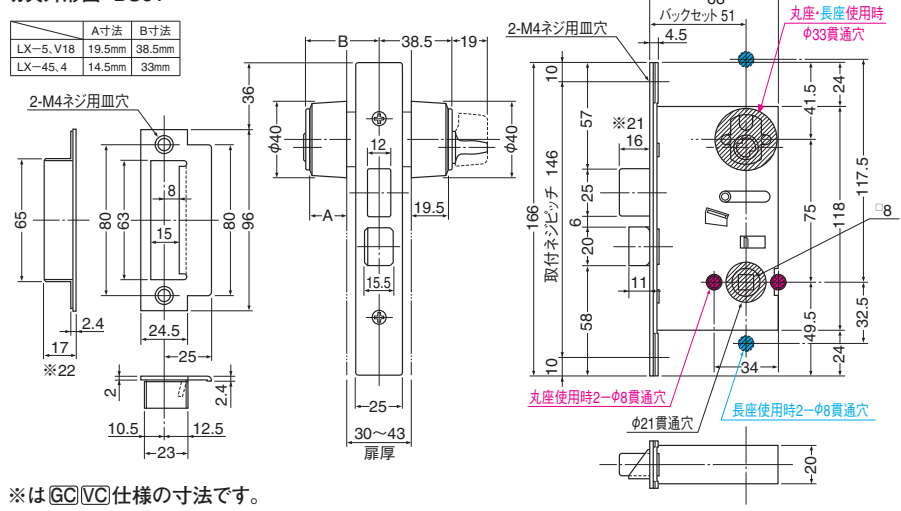
切欠外形図 BS51
