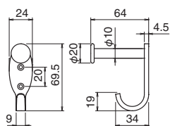
CF-30 クララ帽子掛 (鉄/3.1×22)
