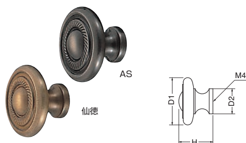
KB-57 マドレーヌツマミ (真チュウ/ISO4×28)
