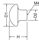
ST-64 ステンキノコツマミ (ステンレス/4×28)
