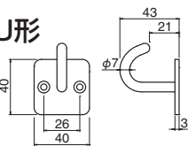
ST-265 ステンダエンフックU形 (ステンレス/A4×25)
