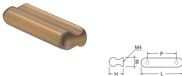
KB-48 ブロンツマミ (真チュウ/ISO4×28)
