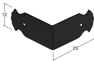
LA-3 エル 黒 110 12×25×25 600個入
