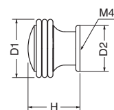
KB-64 イーグルツマミ (真チュウ/ISO4×28)
