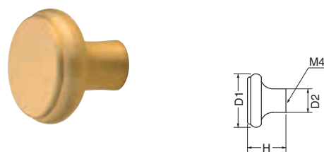
KB-80 アベニューツマミ (真チュウ/ISO4×28)
