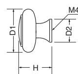
ST-66 ステンクラシカツマミ (ステンレス/4×28)
