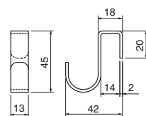
ST-90 長押フック (ステンレス)
