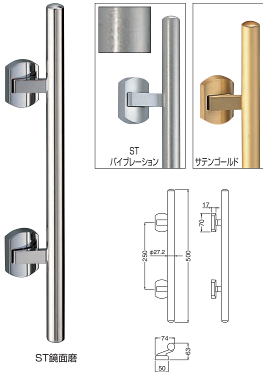
SPP-6 甲丸丸棒 (ステンレス、真チュウ)
