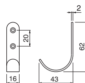
ST-57 ステン小判J形フック (ステンレス/3.1×16)
