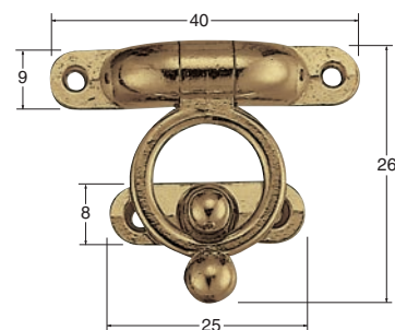
LA-72 UFO前金具 純金 1,300 100個入
