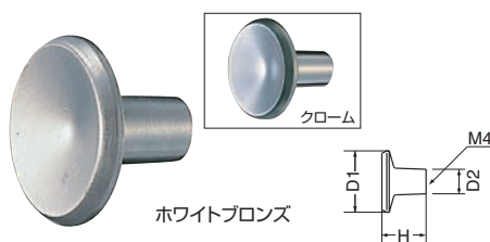
KZ-8 円月ツマミ (亜鉛合金/ISO4×28)
