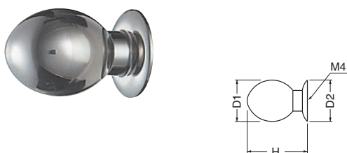
ST-78 ステンどんぐりツマミ (ステンレス/4×28)
