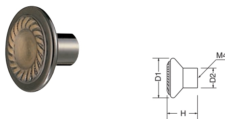
KB-18 ミュンヘンツマミ (真チュウ/ISO4×30)
