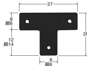
LA-4 T字形 黒 20×27 70 細 20×27 70 1,000個入
