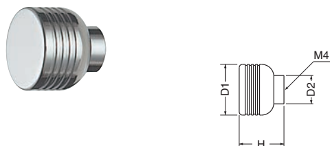
ST-76 ステンマゼランツマミ (ステンレス/4×28)
