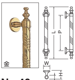
No.40 グラナダ取手 木ネジ止め (真チュウ/3.1×22)
