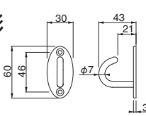
ST-265 ステンダエンフックU形 (ステンレス/A4×25)
