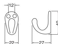
CB-8 唐草フック (真チュウ/3.1×22)
