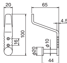
CF-29 アラムス帽子掛 (鉄/3.1×22)
