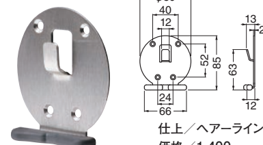
FEX-5 ステン消火器フック丸形 (ステンレス+エラストマー/A4×25)
