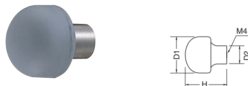
G-10 ゴムマロンツマミ (ゴム+真チュウ/ISO4×28)
