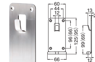
FEX-1 PAT. ステン消火器フックB形 (ステンレス+エラストマー/A4×25)
