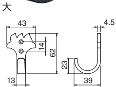
CF-20 リップルフック (鉄/3.1×16)
