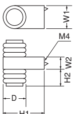
KB-70 マルシェツマミ (真チュウ/ISO4×28)
