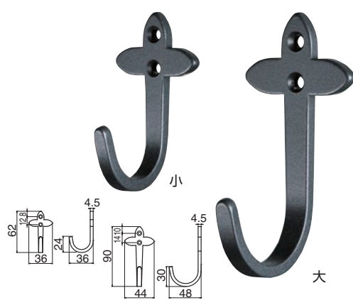
CF-16 アンティークフックローバー (鉄/3.1×16)
