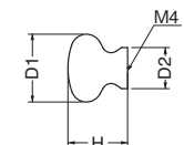
KW-24 ウッドアスターツマミ (積層/ISO4×28)
