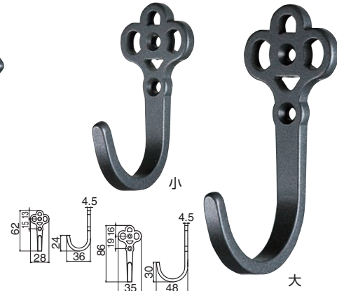
CF-19 アンティークフックカメラ (鉄/3.1×16)
