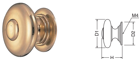
KB-58 マイヨーツマミ (真チュウ/ISO4×28)
