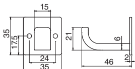
ST-291 ステンフラットフック (ステンレス/A4×25)
