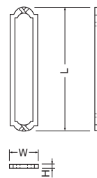
No.11P スパニッシュ押板 木ネジ止め (真チュウ/3.5×25)
