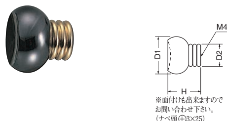
KB-61 ミラージュツマミ (真チュウ/ISO4×28)
