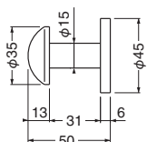
CW-1 キノコフック (積層/3.1×22)
