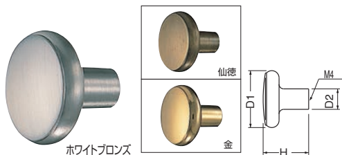
KZ-22 カスタムツマミ (亜鉛合金/ISO4×28)
