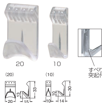
PAT. Uピンタイプ C-100 ラインフック (ポリカーボネート)
