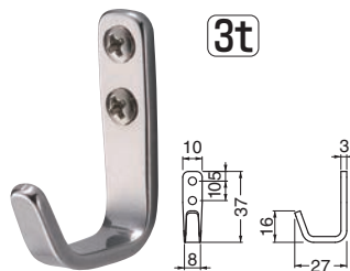
ST-251 ステン角J形フック (ステンレス/低頭A3×16)
