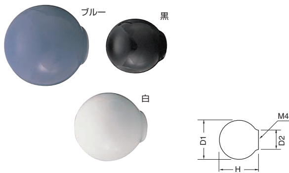
KT-1 セラミックボールツマミ (セラミック/ISO4×28)
