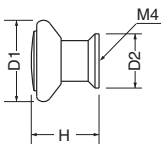
KB-50 シャモニツマミ (真チュウ/ISO4×28)
