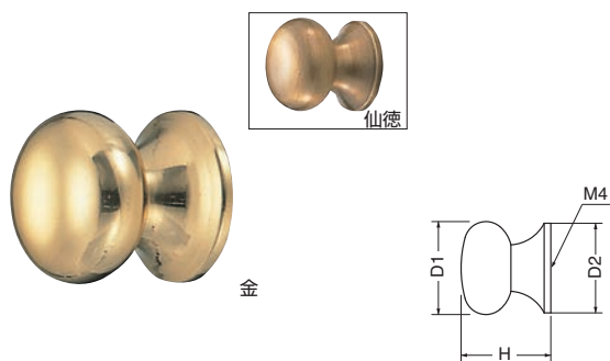
KB-56 モンブランツマミ (真チュウ/ISO4×28)
