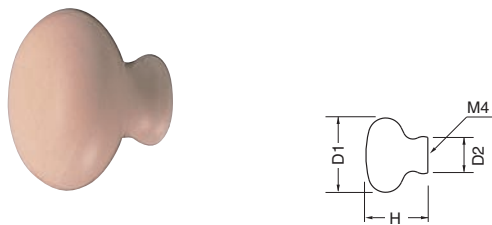
KT-2 セラミックアーモンドツマミ (セラミック/ISO4×28)
