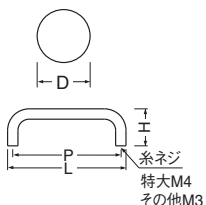
HB-100 真チユウ100番丸棒ハンドル (真チユウ)
