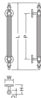
No.36 バルカン取手 木ネジ止め
