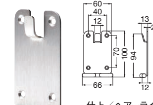
FEX-3 PAT. ステン消火器フックU形 (ステンレス+エラストマー/A4×25)
