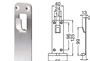
FEX-2 PAT. ステン消火器フックスリム形 (ステンレス+エラストマー/A4×25)
