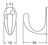
CZ-10 コート掛 (亜鉛合金/2.7×16)
