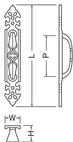
No.10 スパニッシュ座付取手 木ネジ止め (真チュウ/3.5×25)
