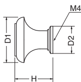
KB-59 アルバツマミ (真チュウ/ISO4×28)
