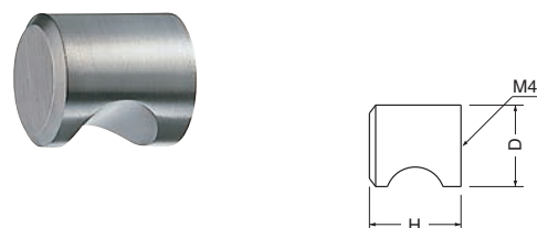
ST-14 ステン面取円筒ツマミ (ステンレス/NL4×28)
