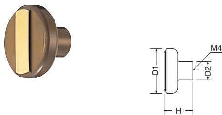
KB-35 オリビアツマミ (真チュウ/ISO4×28)
