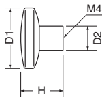
ST-61 ステン甲丸ラウンドツマミ (ステンレス/4×28)
