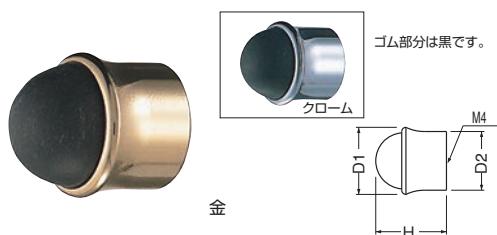
G-12 バウンドツマミ (ゴム+真チュウ/ISO4×30)
