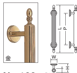
No.103 コルドバ取手 木ネジ止め (真チュウ/3.1×22)
