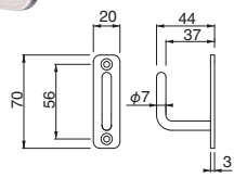
ST-266 ステン角形フックL形 (ステンレス/A4×25)
