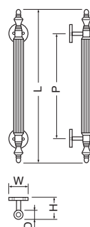
No.64 プチバルカン取手 木ネジ止め
