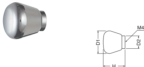
ST-82 ステンアニーツマミ (ステンレス/4×28)
