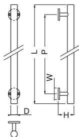
No.68 丸型取手 木ネジ止め
