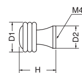
KB-76 ドリアツマミ (真チュウ/ISO4×28)
