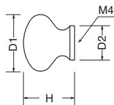
KW-16 ボローニヤツマミ (自然木/ISO4×28)
