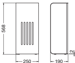
FEX-101 消火器スタンドB形 (ステンレス)
