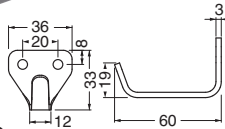
ST-260 ステンソアラフック (ステンレス/低頭A4×25)
