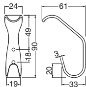
ST-280 ステンダ・ヴィンチ帽子掛L形 (ステンレス/低頭A4×25)
