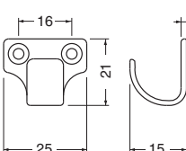
CB-21 デルタフック (真チュウ、ステンレス/3.1×16)
