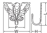
CB-9 タカフック (真チュウ/3.1×22)
