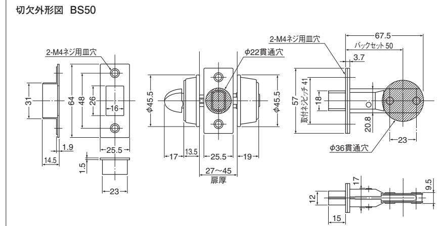
切欠外形図 BS50
