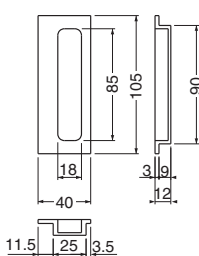
MW-18 ウッドリアル戸引手 (積層)
