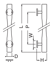
No.21 ウッド杵形取手 木ネジ止め (横溝+真チュウ/3.1×22)
