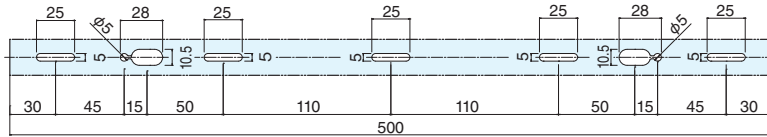
共通取付穴 詳細図
