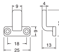
CB-20 T形フック (真チュウ/3.1×16)
