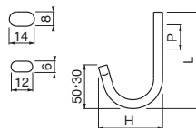
ST-50 ステンJ形フック (ステンレス/3.5×22)
