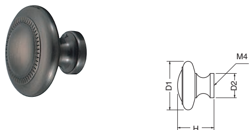
KB-51 オデオンツマミ (真チュウ/ISO4×28)
