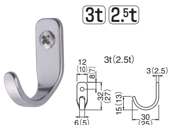
ST-250 ステンミニJ形フック (ステンレス/低頭A3×16)
